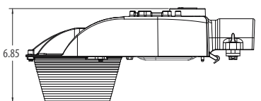
D3/D5 Optic
